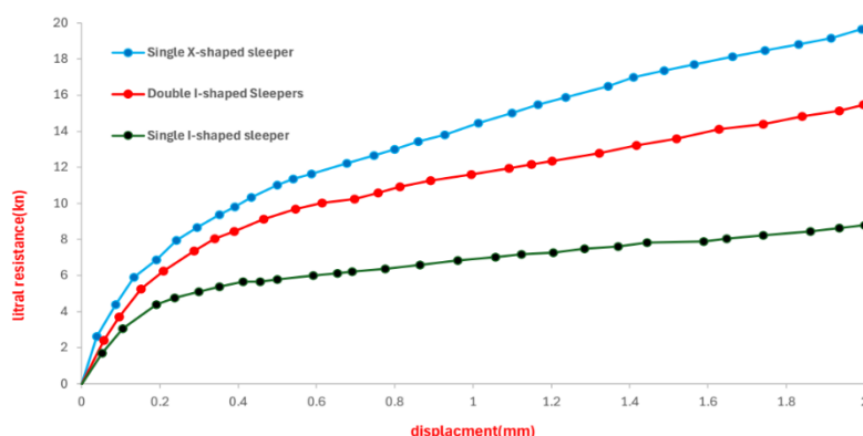
شکل (۹)- نمودار مربوط به مقایسه تراورس X شکل با I شکل (Chen et al., ۲۰۲۴)
