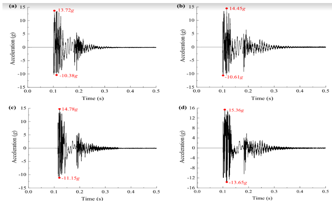
شکل (۴)- شتاب ارتعاش تراورس در حوزه زمان (Liu et al., ۲۰۲۳)
