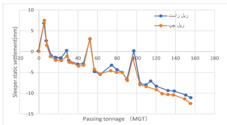
شکل (۶)- تغییر نشست استاتیکی تراورس با بارهای مکرر قطار (Ishida & Makoto, ۲۰۱۵)
